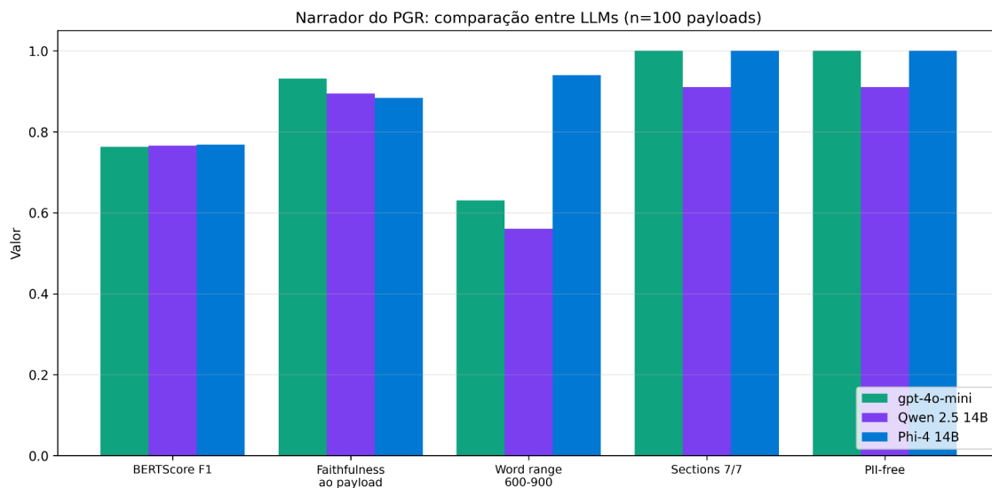
Figura 10 - Narrador do PGR, métricas primárias (3 modelos)
