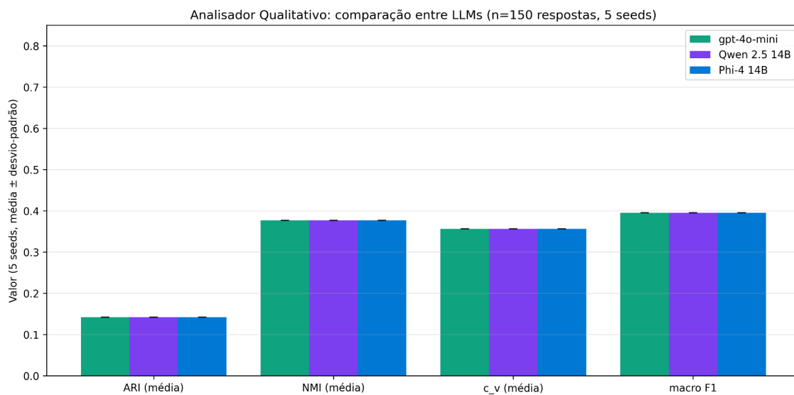
Figura 11 - Analisador qualitativo, ARI/NMI/c_v/F1 (3 modelos, 5 seeds)
